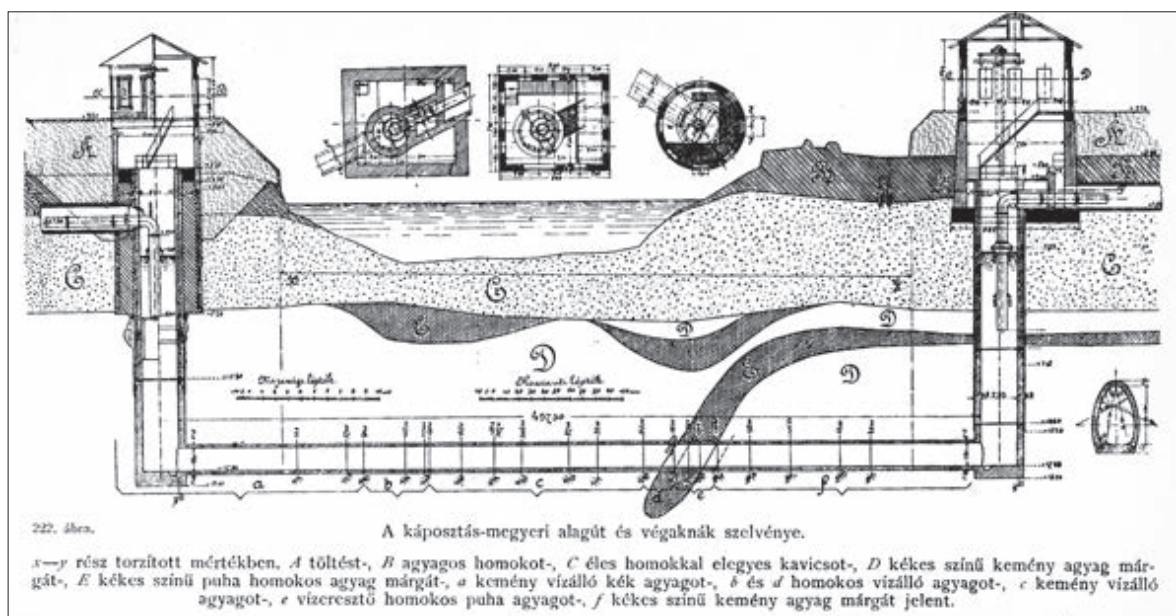
A főtelep szifonjának jellemző keresztmetszete a tojásszelvényű (vízvezeték) alagúttal, a kútházakkal, a jellemző talajszelvényekkel és kútház alaprajzokkal
