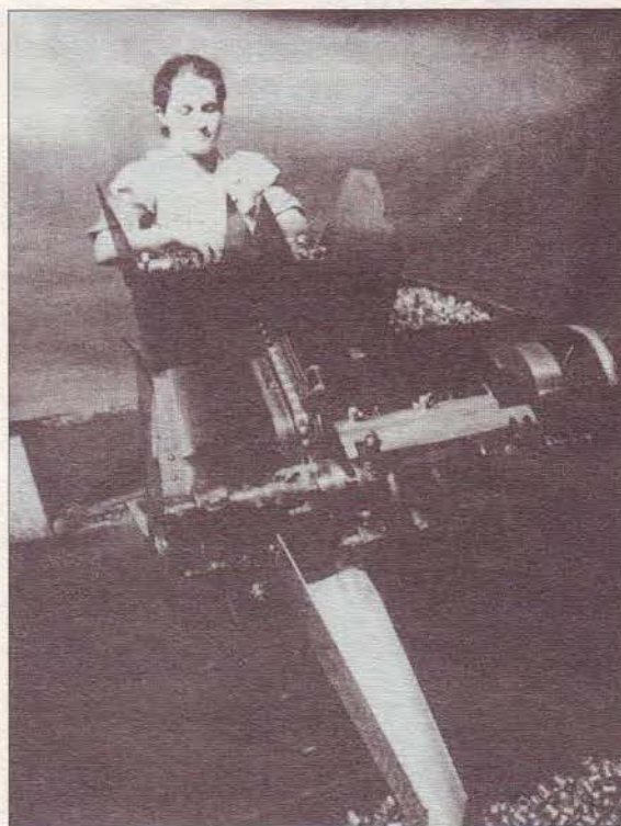
Kéziadagolású menetmángorló gép a lámpafénygyártásban, 1910-es évek vége, 1920-as évek eleje
