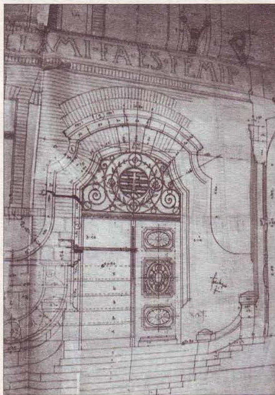
Foerk Ernő eredeti kaputerve
